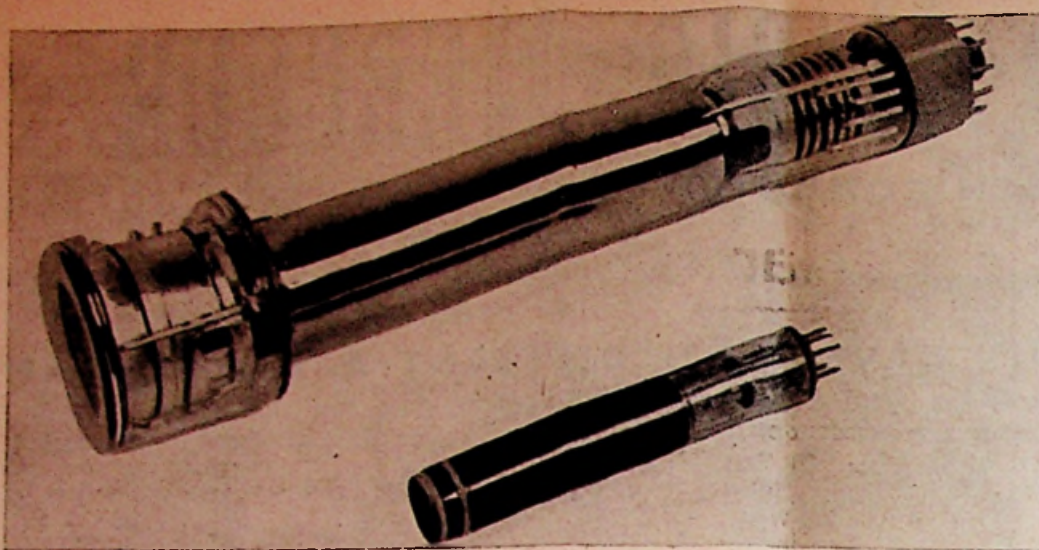
Een vergelijking in grootte tussen twee opnamebuizen voor televisie voor gelijke gevoeligheid: boven de image-orthicon met ingebouwde electronenvermenigvuldiger; onder de Vidicon.
